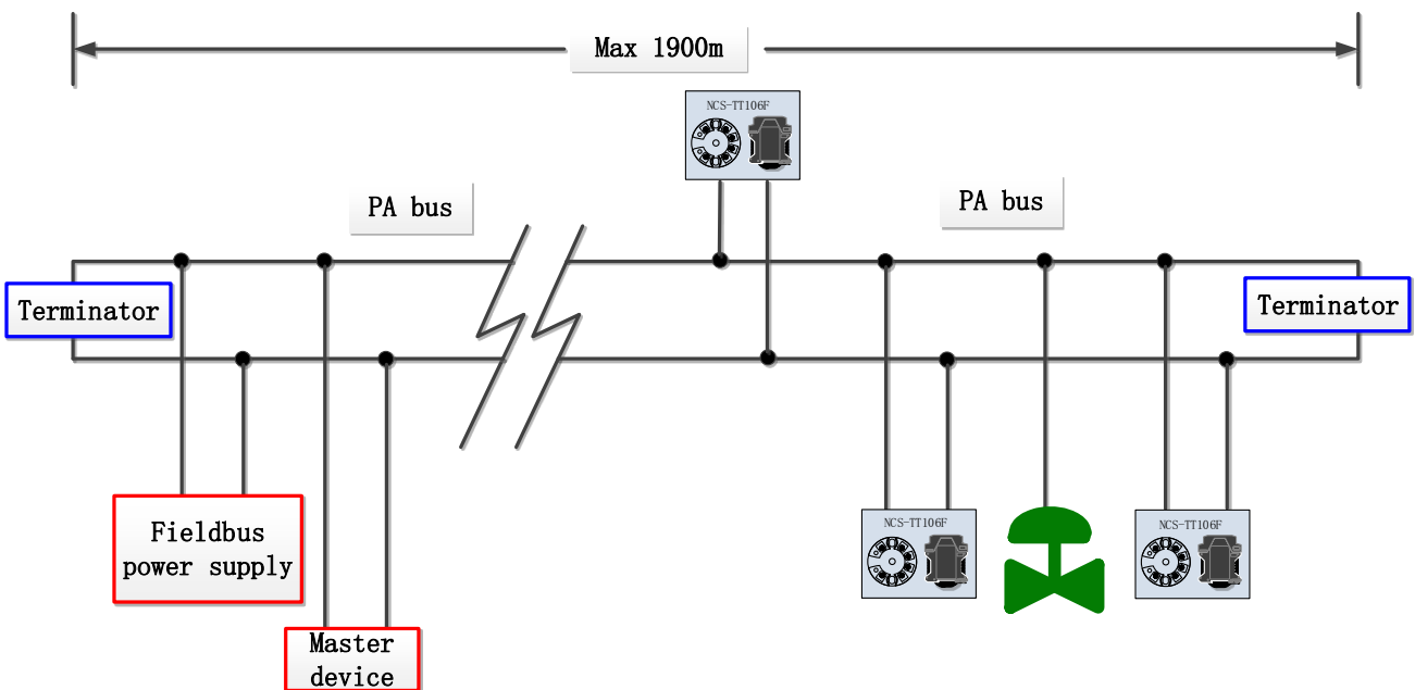
Figure 错误!文档中没有指定样式的文字。 .5 PROFIBUS PA bus connection
