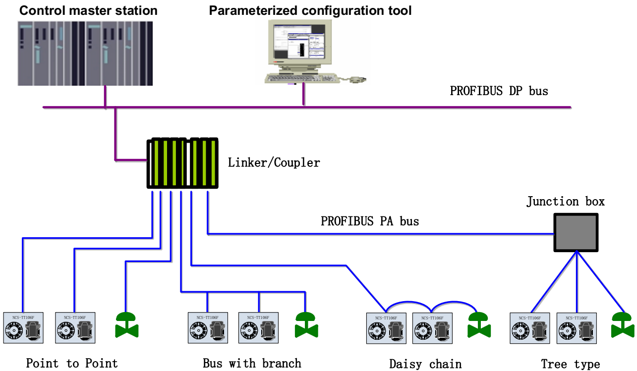
Figure 错误!文档中没有指定样式的文字。 .4 PROFIBUS PA network topology
