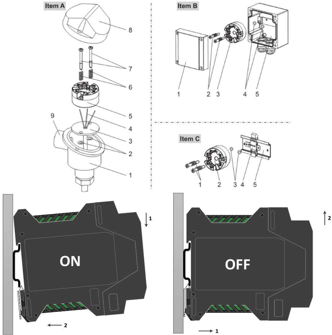
Figure 错误!文档中没有指定样式的文字。 .2 Installation
